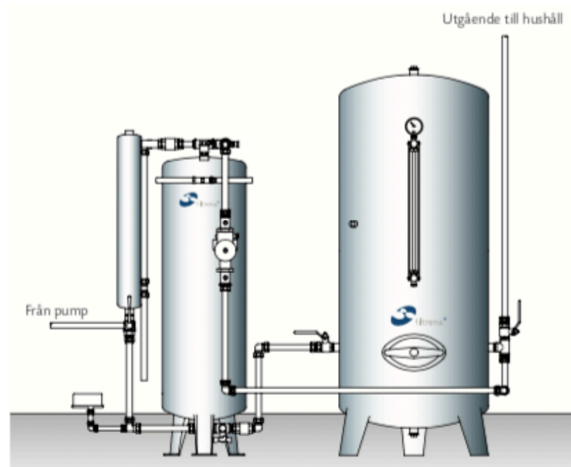
Installationsskiss
